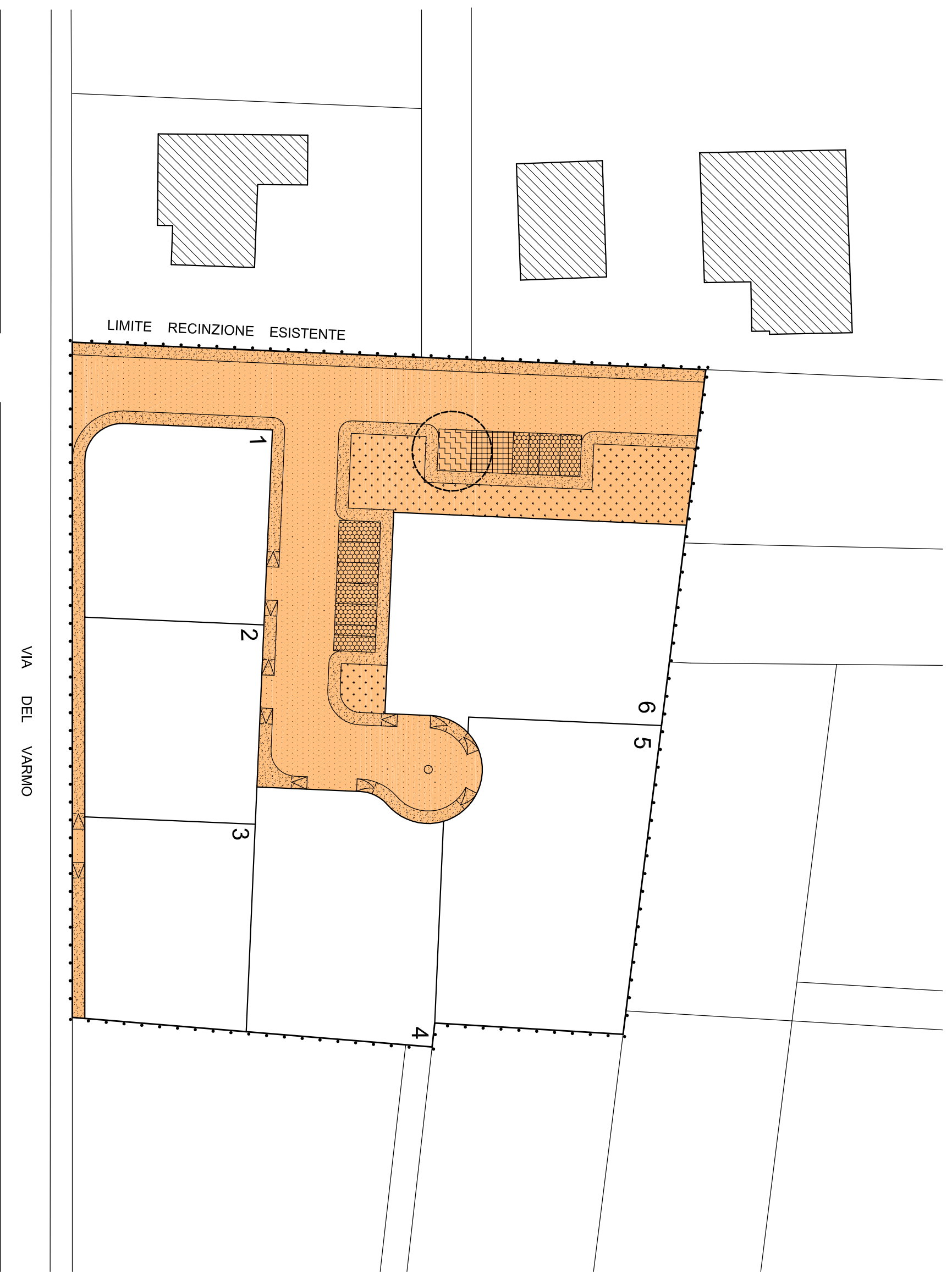
PIAZZOLA RACCOLTA RIFIUTI - Scala 1:100
